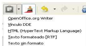
Figura 9: Menú Pegar
